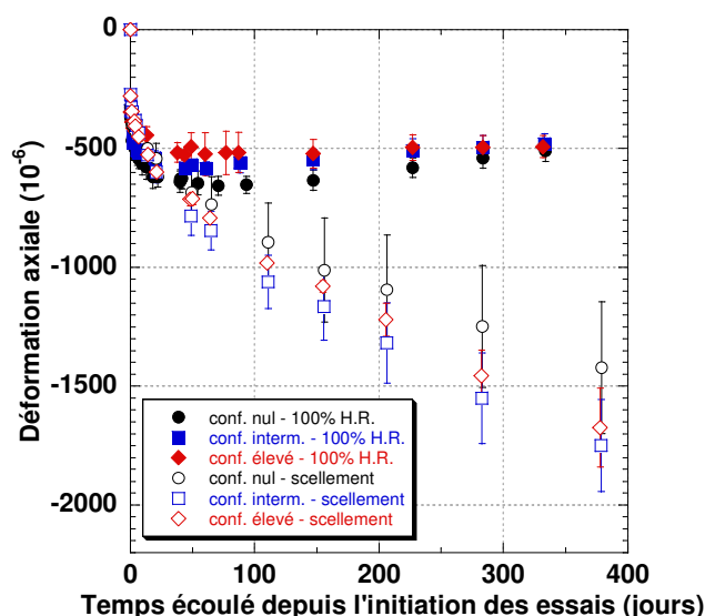
FIGURE 7 Évolution comparative des déformations axiales dans les éprouvettes soumises à un chargement soutenu de 10 MPa en fonction des conditions d'exposition hygrométriques (100% H.R. vs scellement) et du niveau de confinement latéral (nul, intermédiaire, élevé).
