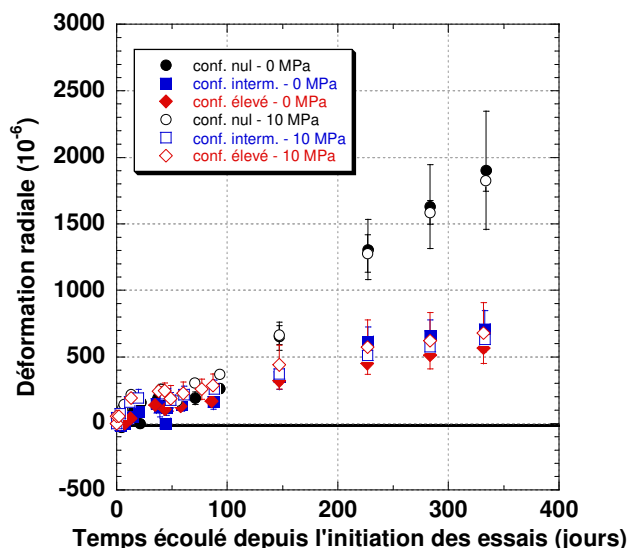
FIGURE 8 Évolution comparative des déformations radiales dans les éprouvettes non chargées et chargées (10 MPa) exposées à 100% H.R. en fonction du niveau de confinement latéral (nul, intermédiaire, élevé).
