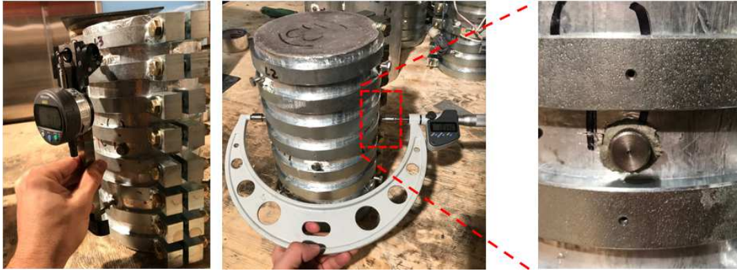
FIGURE 3 Disposition des plots et extensomètres utilisés pour la mesure des déformations axiales et radiales
