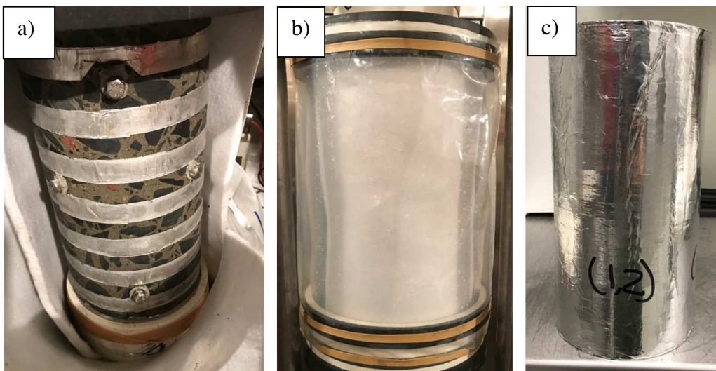
FIGURE 2 Conditions hygrométriques des éprouvettes: a) éprouvette exposée à 100% H.R. avec l'enceinte ouverte; b) éprouvette à 100% H.R. avec l'enceinte fermée; c) éprouvette scellée.
