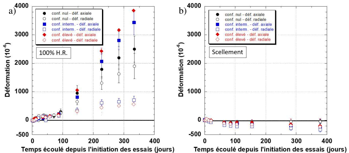
FIGURE 4 Évolution des déformations dans les éprouvettes non chargées axialement en fonction du niveau de confinement latéral (nul, intermédiaire, élevé): a) à 100% H.R.; b) en conditions scellées.
