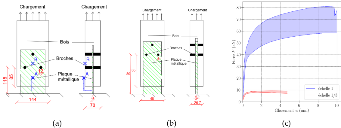
FIGURE 1. Essais réalisés, a : montage à l'échelle 1, b : montage à l'échelle 1/3, c : courbes force – glissement (fuseau) pour les deux échelles
