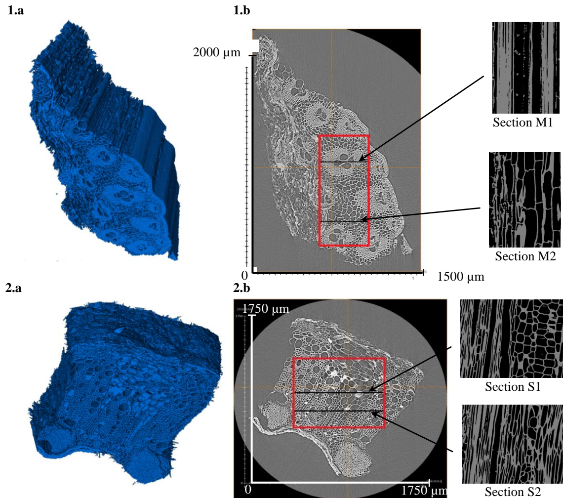
Figure 2. Volume 3D reconstitué (a) et images de sections transversales (b) de particules d'écorce de maïs (1) et de tournesol (2) obtenues par tomographie à rayons X (les écorces sont en gris sur les sections M1, M2, S1, S2).
